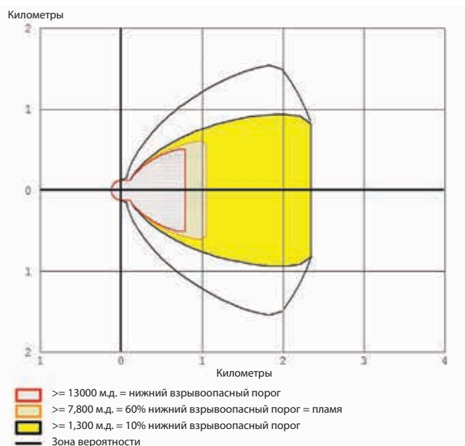
▲ Рис. 12: Различные критические уровни (взрывоопасности) для циклогексана в зависимости от расстояния до источника возгорания; показано на примере выходных данных модели ALOHA Национального управления океанических и атмосферных исследований США. ALOHA = Area Locations of Hazardous Atmospheres (расположение зон с опасными условиями).
