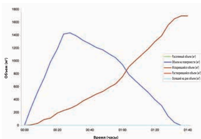
Рис. 13: Пример модели поведения утечки конечного объема циклогексана (C6H12) с борта затонувшего судна, в динамике по времени. Как показывают кривые на графике, циклогексан поднимается к поверхности воды и постепенно испаряется в атмосферу. Площадь разлива достигнет максимальных размеров через 20 часов с момента аварии. Циклогексан является несмешиваемым веществом с плотностью 0,78 г/см³, поэтому уровни его растекновения, осаждения на морское дно и рассеивания являются незначительными или близкими к нулю (источник: компания Chemsys — Национальный центр по ликвидации и предотвращению химических катастроф (NCEC), http://the-ncec.com ).
